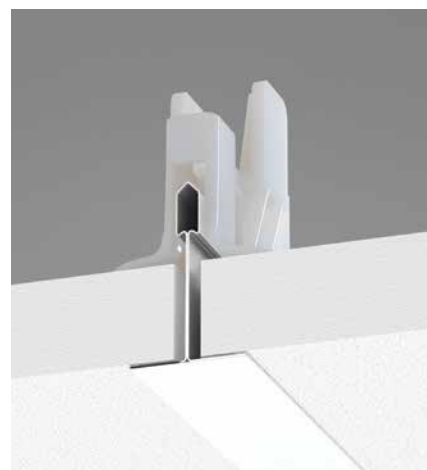
Figur 11. Absorbent i skinnesystem monteret med clips, nedhængt fra loft nedhængt
